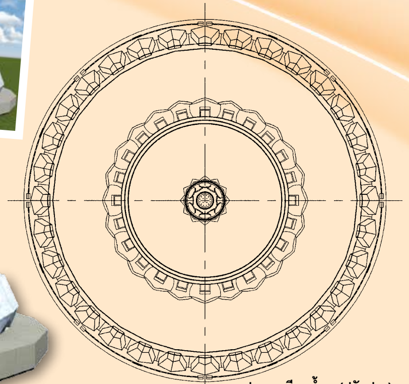
แปลนวงเวียนน้ำพุ (ปรับปรุง)
